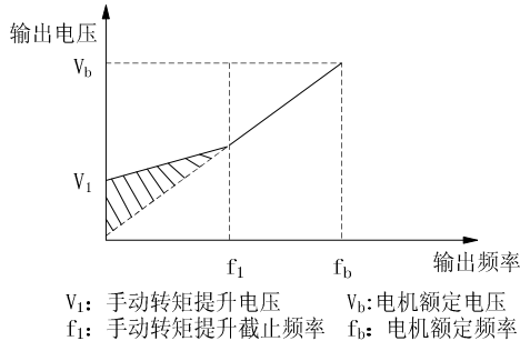
图 6-6 手动转矩提升示意图
