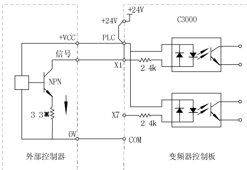
图 4-11 漏型接线方式
