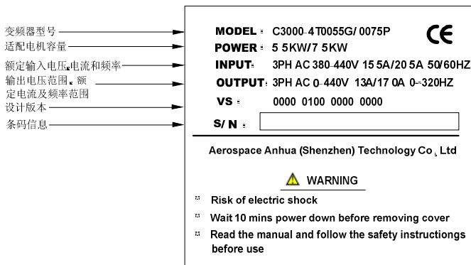
图 3-2 C3000 变频器铭牌
