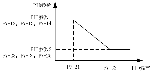
图 6-17 PID 参数切换
