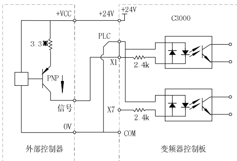
图 4-13 源型接线方式
