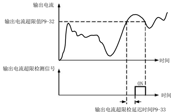
图 6-23 输出电流超限检测示意图
