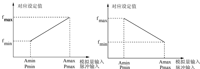
图 6-12 模拟/脉冲给定与设定量的对应关系
