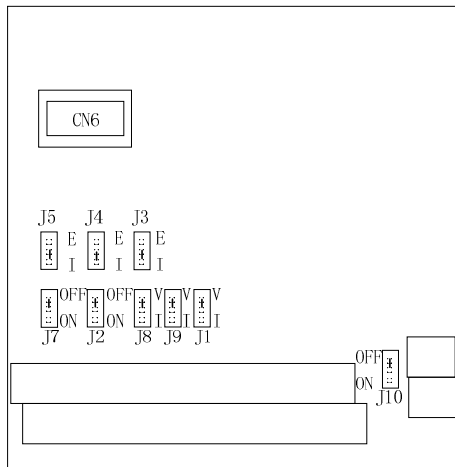
C3000-4T0055G/0075P 以上 图 4-8 控制板的跳线开关位置示意图
