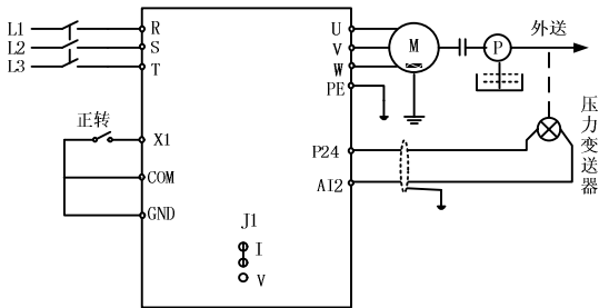
图 10-4 外部端子和电流型压力反馈接线图
