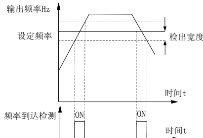
图 6-13 频率到达检出幅值示意图
