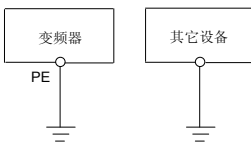
图 4-18 接地示意图 1
