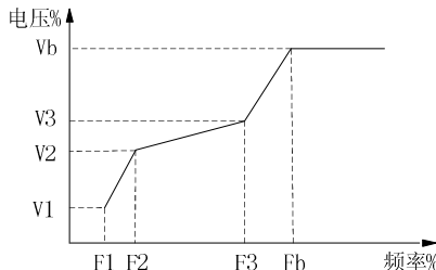
V1~V3：多段速V/F第1~3段电压百分比 F1~F3：多段速V/F第1~3段频率百分比 Vb：电压额定电压 Fb：电机额定运行频率
