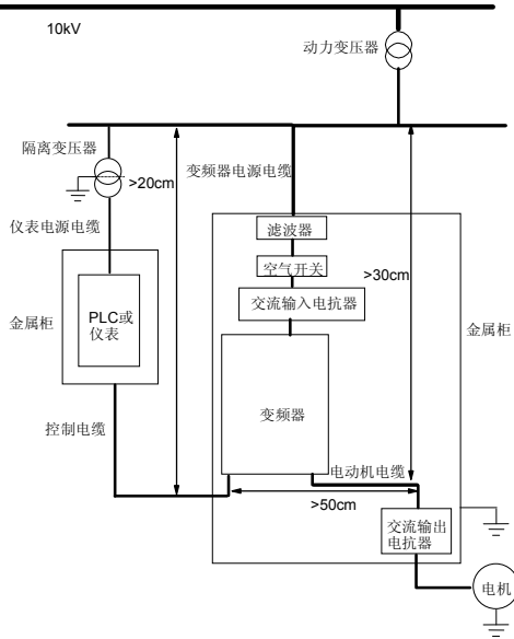
图 4-5 变频器的安装示意图
