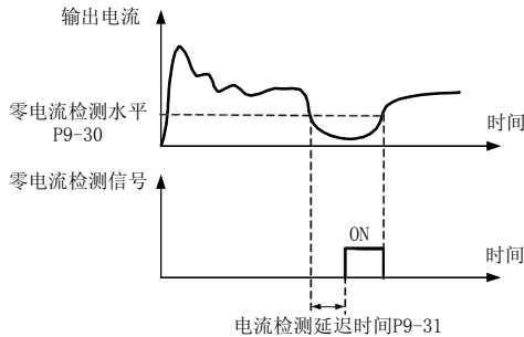
图 6-22 零电流检测示意图
