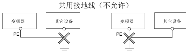
图 4-20 接地示意图 3
