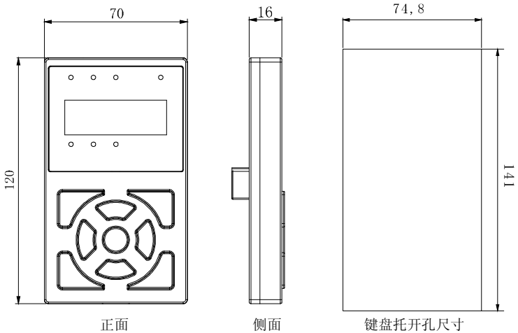
C3000-4T0040G/0055P 及以上的键盘外形尺寸
