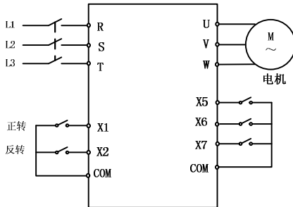
图 10-2 外部端子和多段速控制接线图
