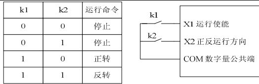
图 6-9 两线式模式 2
