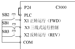
图 6-10 三线式控制模式 1
