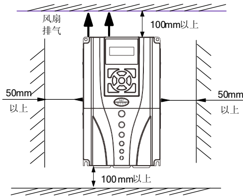
图 4-1 安装的间隔距离
