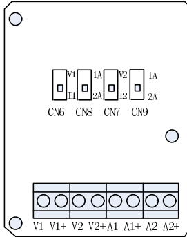
图 1 注塑机扩展卡的跳线开关位置示意图
