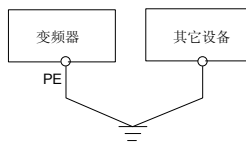
图 4-19 接地示意图 2
