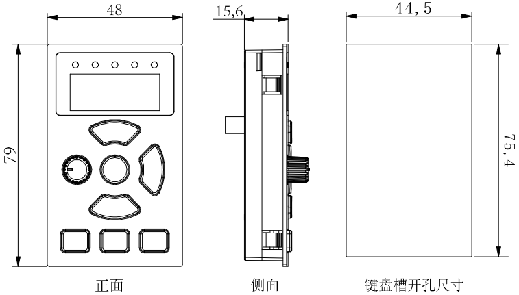
C3000-2S0004G~4T0022G 的键盘外形尺寸
