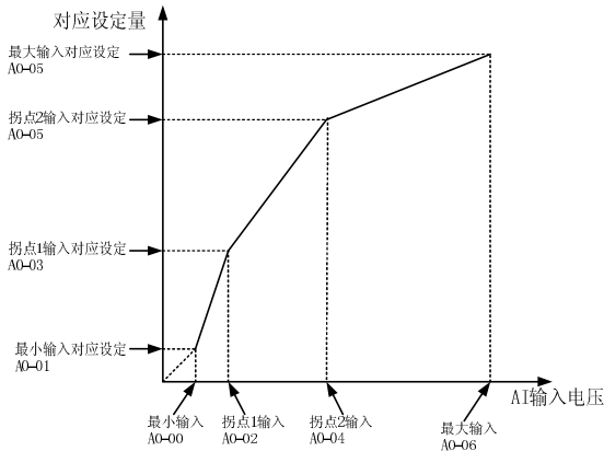
图 6-30 曲线 4 示意图
