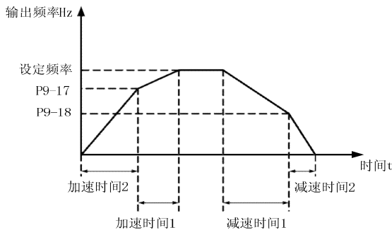
图 6-21 加减速时间切换示意图
