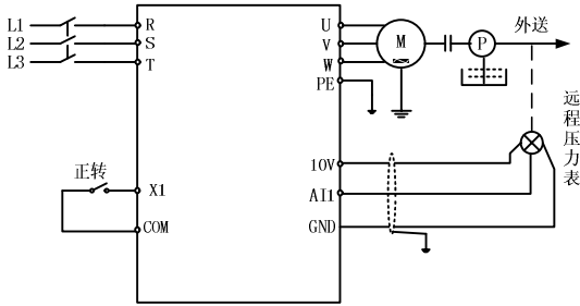
图 10-3 外部端子和电压型压力反馈接线图
