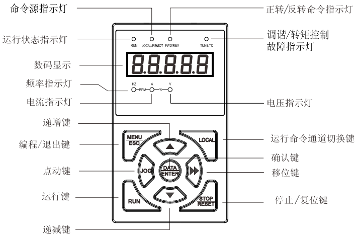
图 5-1 C3000-4T0040G~C3000-4T800G LED 操作面板示意图
