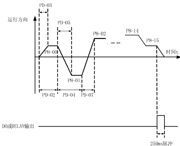
图 6-26 简易 PLC 示意图
