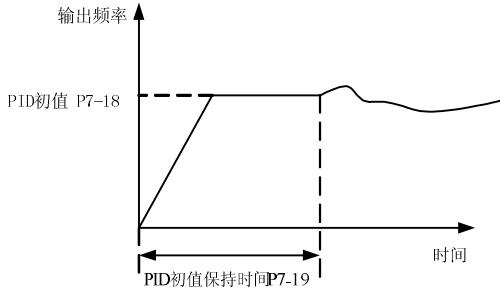
图 6-16 PID 初值功能示意图
