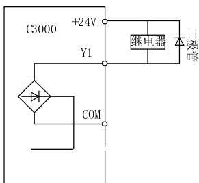
图 4-14 数字输出端子接线示意图
