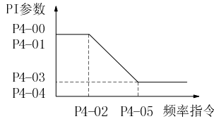
图 6-7 PI 参数示意图
