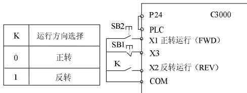
图 6-11 三线式控制模式 2
