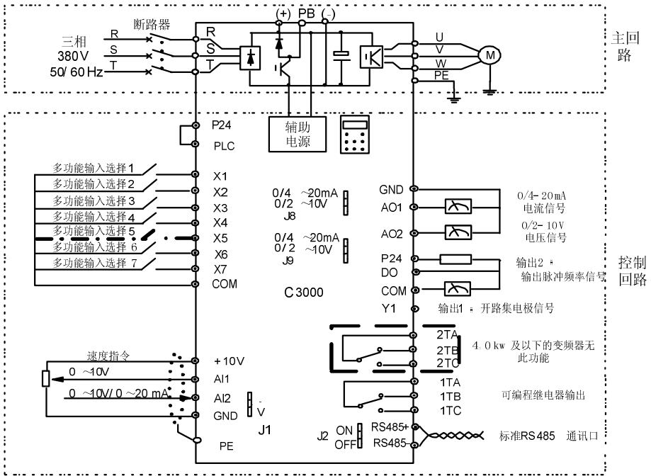
图 4-7 基本配线图
