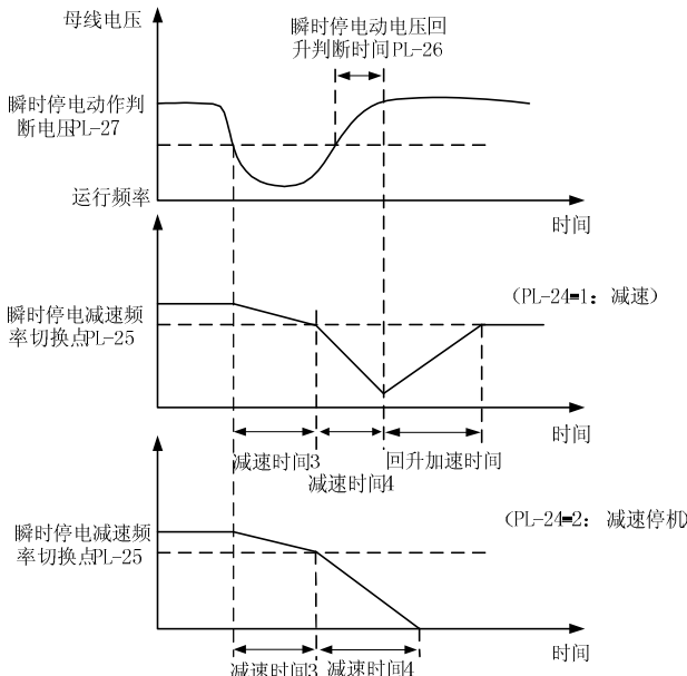
图 6-29 瞬时停电动作示意图
